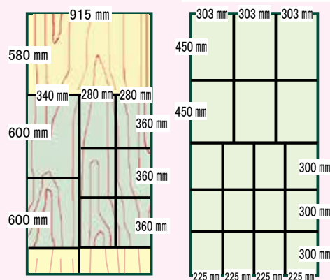
特注カット図面例
